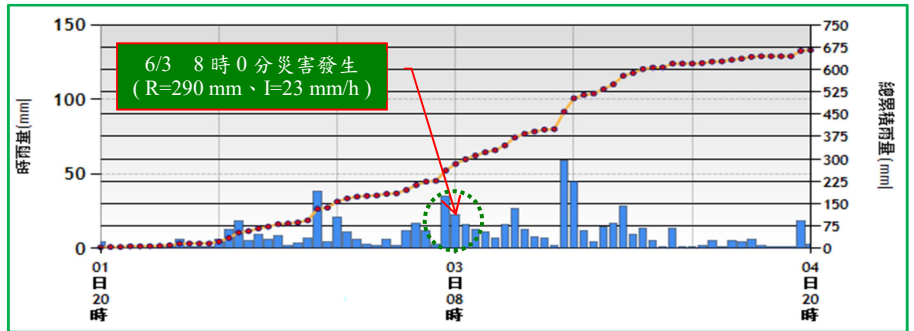
(參考雨量站：鯉潭 (C1125) 土石流警戒基準值：300mm)
