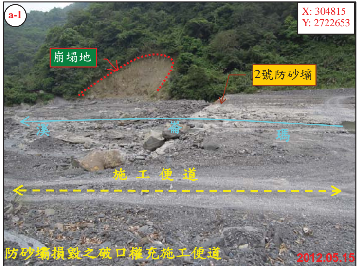
水保局辦理瑪崙溪災害防治四期工程 2012.05.15
