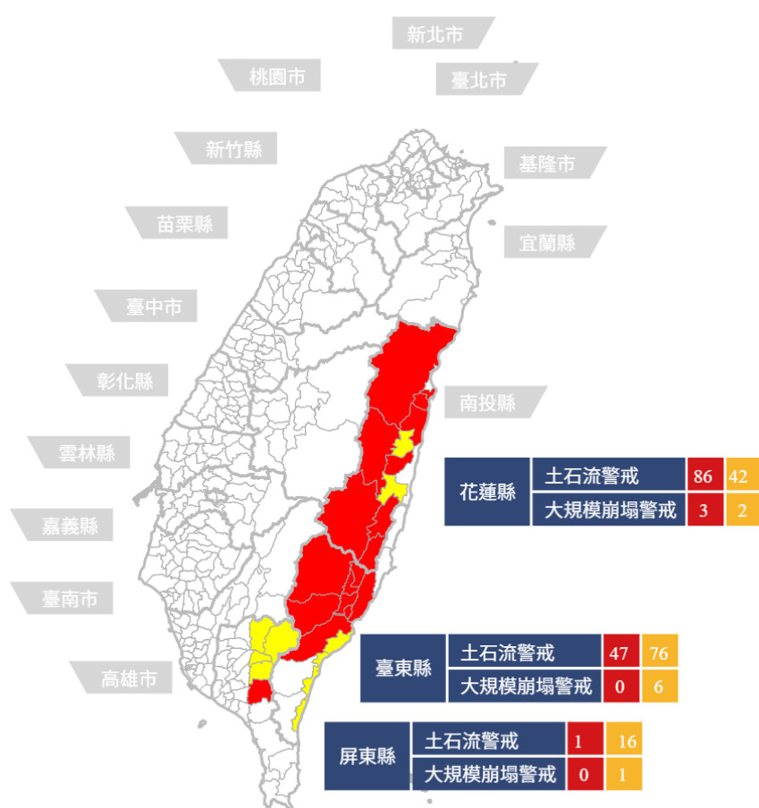
圖 1-1 114 年樺加沙颱風土石流及大規模崩塌警戒發布空間分布(最大發布數量 9/24 12:30 第 13 報)
