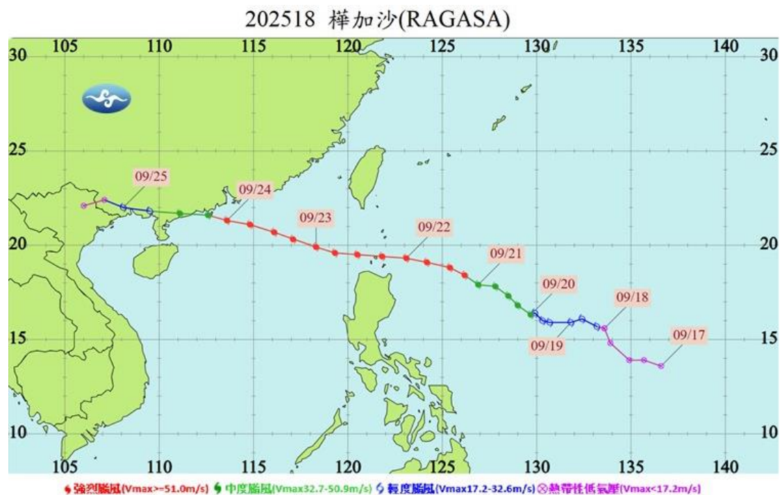
圖 1-3 樺加沙颱風路徑圖
