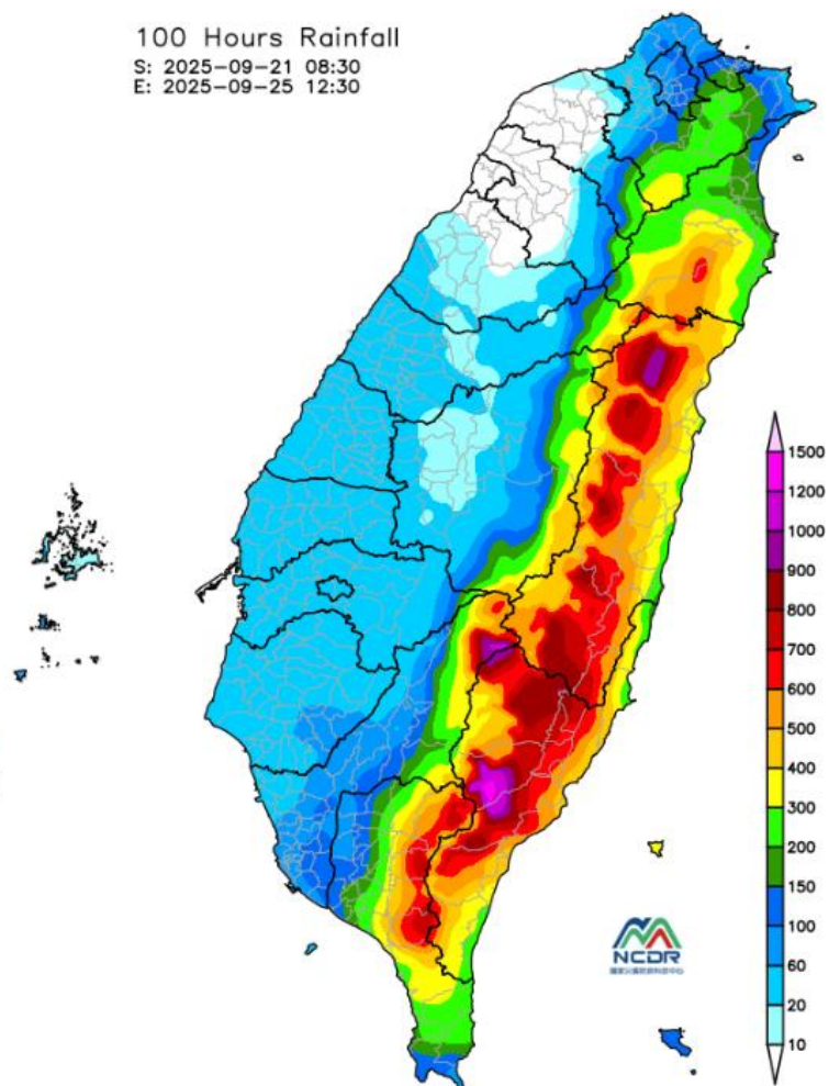
圖 1-2 114 年樺加沙颱風累積雨量空間分布
