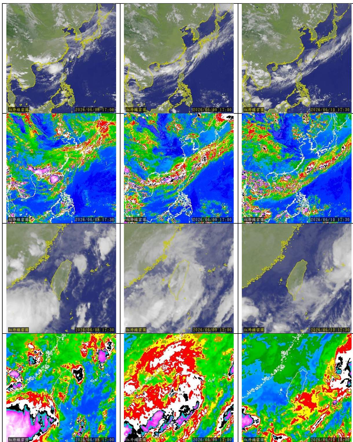
圖 1-3 115 年 0608 豪雨衛星雲圖
