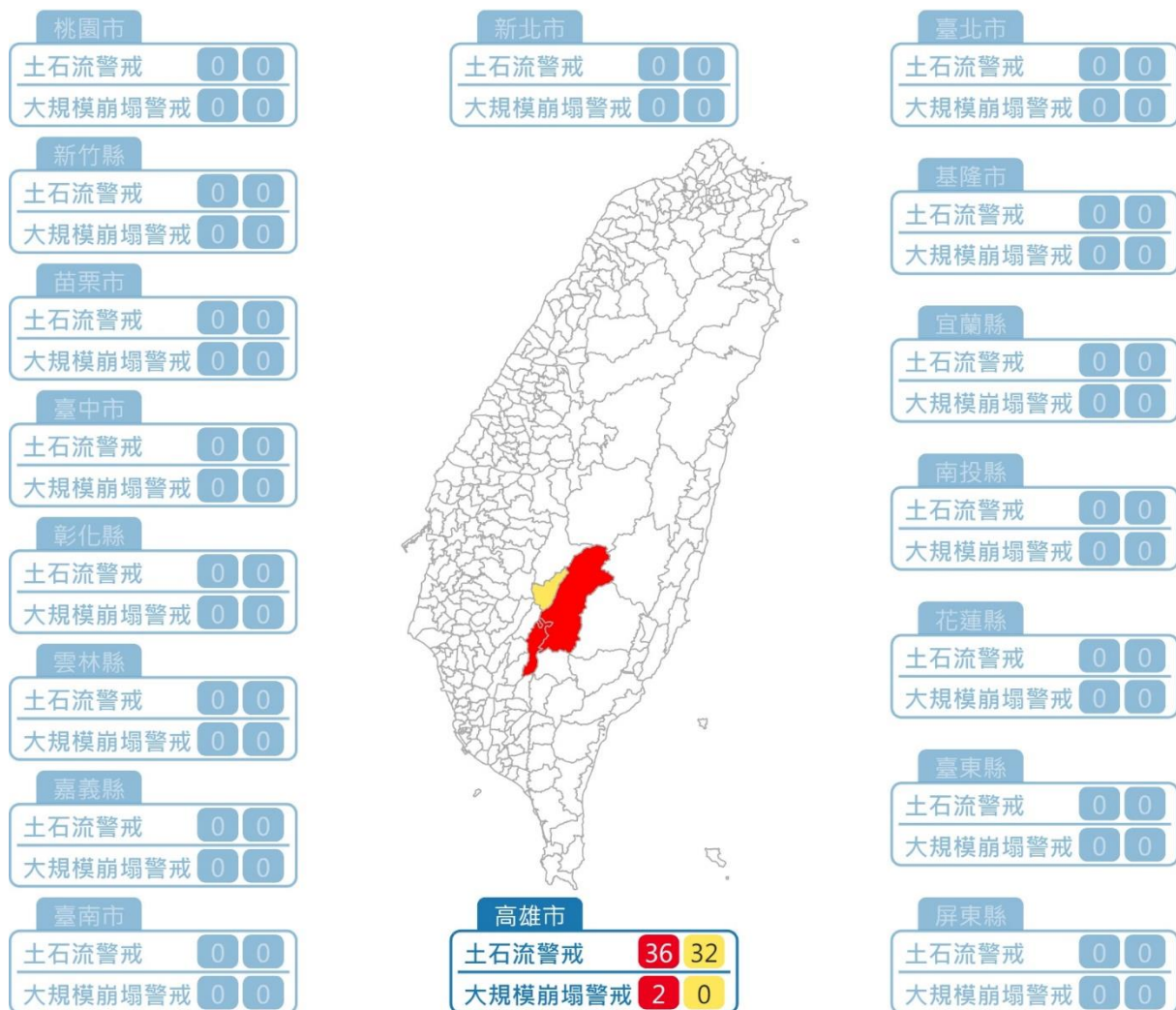
圖 1-1 115 年 0608 豪雨土石流及大規模崩塌警戒發布空間分布(最大發布數量 06/10 06:30 第 10 報)
