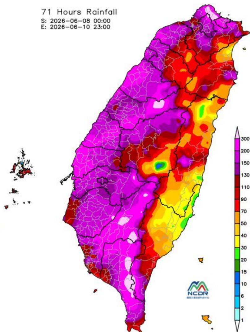
圖 1-2 115 年 0608 豪雨累積雨量空間分布
