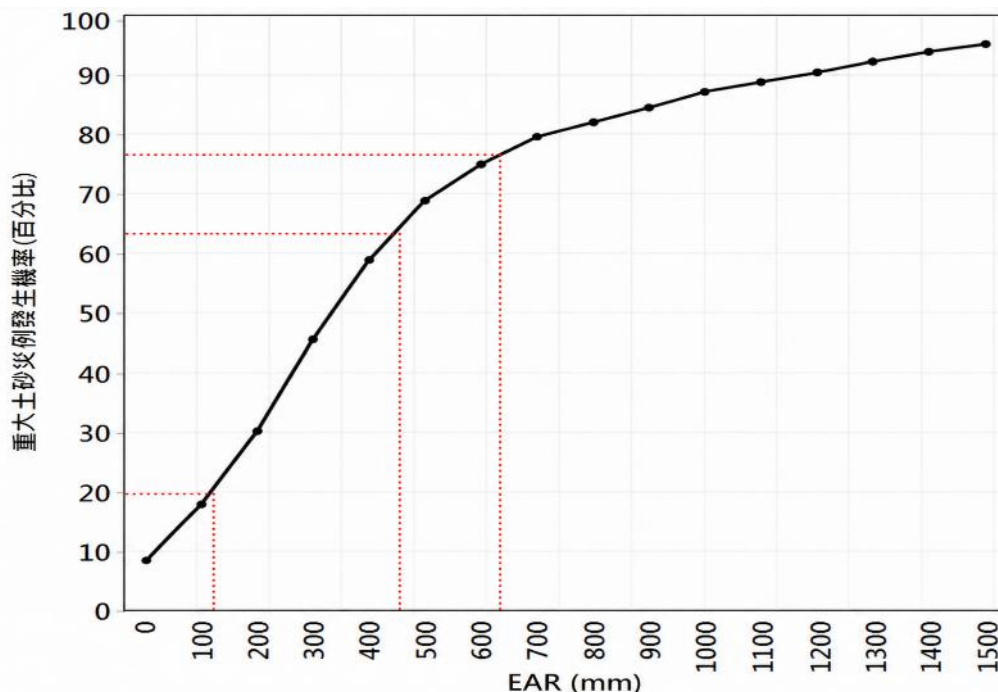
2006-2025重大土砂災例與有效累積雨量級距關係
